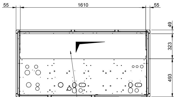
SEZ. A-A
